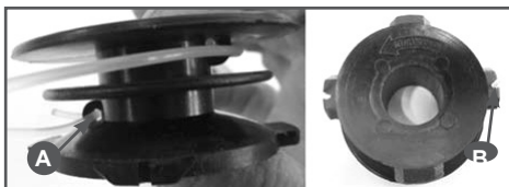
Рис. 24 Установка корда
