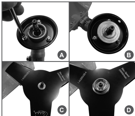
Рис. 4 Установка ножа
