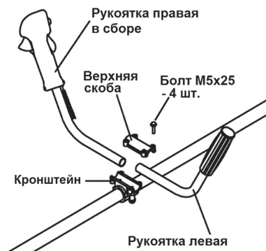
Рис. 6 Установка рукояток
