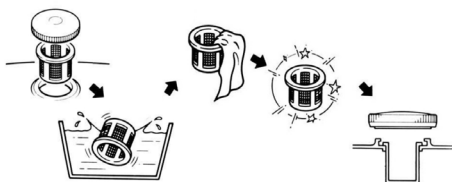
Рис. 18 Обслуживание сетчатого фильтра в горловине топливного бака
