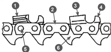
Рис. 27 Конструкция пыльной цепи
